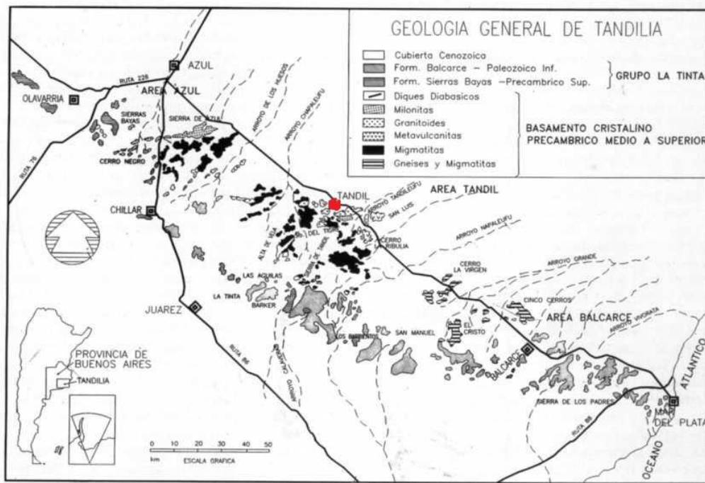
Figura 3. Geología de Tandilia (Dalla Salda et al., 2006).
